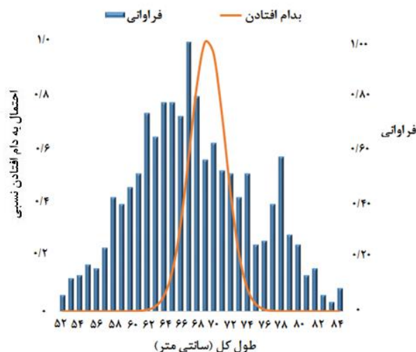
شکل ۶: منحنی انتخاب‌پذیری تور گوشگیر ۱۷ سانتی متر Figure 6: Selectivity curve of gillnet with 17 cm mesh size in relation to L. johni .
