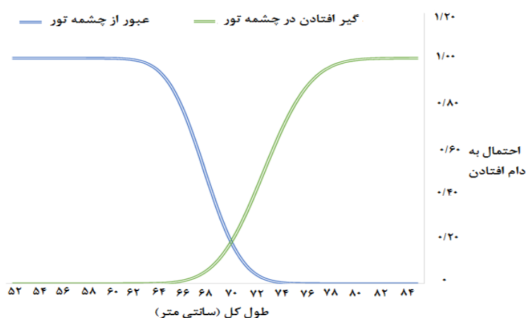
شکل ۵: احتمال به دام افتادن و خروج ماهی سرخو معمولی از تور
