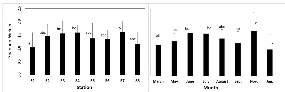
شکل ۲: میانگین شاخص تنوع گونه‌ای شانون-وینر برای ماهیان در ماه‌ها و ایستگاه‌های مختلف رودخانه سفیدرود Figure 2: Average of Shannon-Weiner diversity index for fish in different months and stations of Sefidroud River
