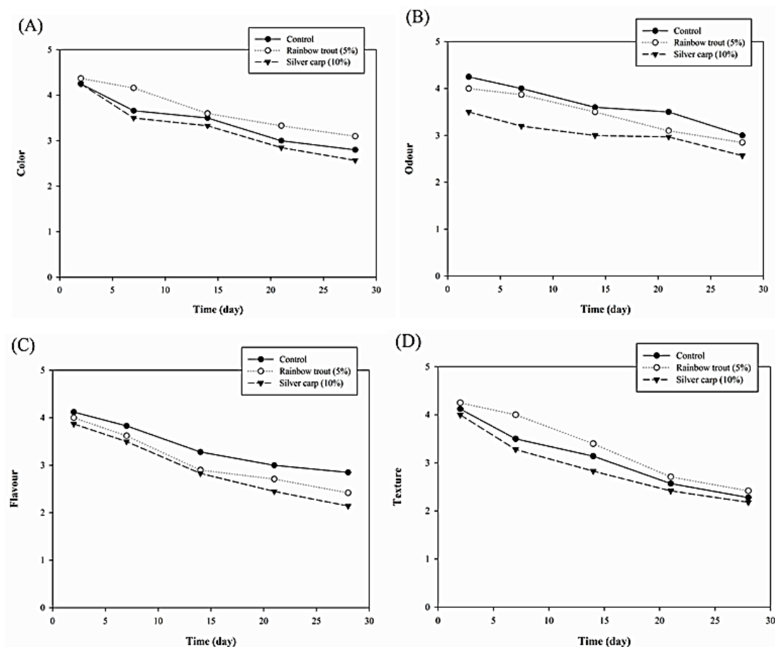
شکل ۲: ویژگی‌های حسی (رنگ (A)، بو (B)، طعم/مزه (C)، بافت (D)) نان‌های فطیر شاهد و غنی شده طی دوره نگهداری در دمای یخچال (۴ درجه سانتی‌گراد)
