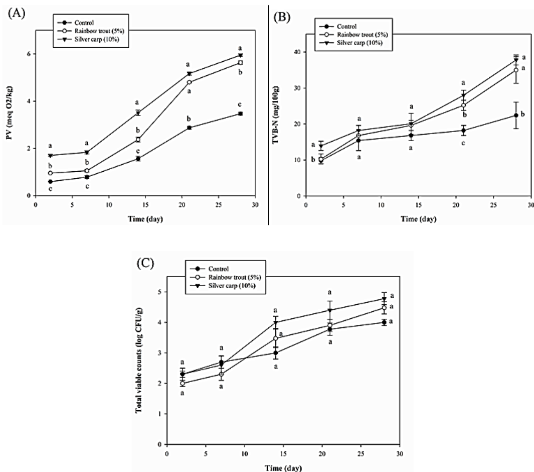
شکل ۱: پراکسید (A)، TVB-N (B) و بار باکتریایی کل (C) نان‌های فطیر شاهد و غنی شده طی دوره نگهداری در دمای یخچال (۴ درجه سانتی‌گراد)
