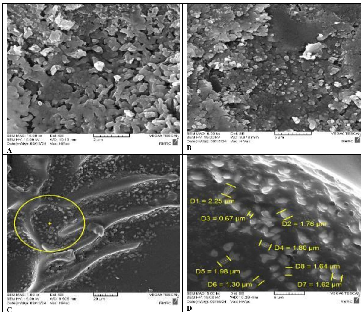
شکل ۱: تصویر میکروسکوپ الکترونی SEM از Lactobacillus plantarum ریزپوشانی شده با ژلاتین-پروتئین هیدرولیز شده ماهی از طریق خشک‌کن انجمادی ( 2000\times )
