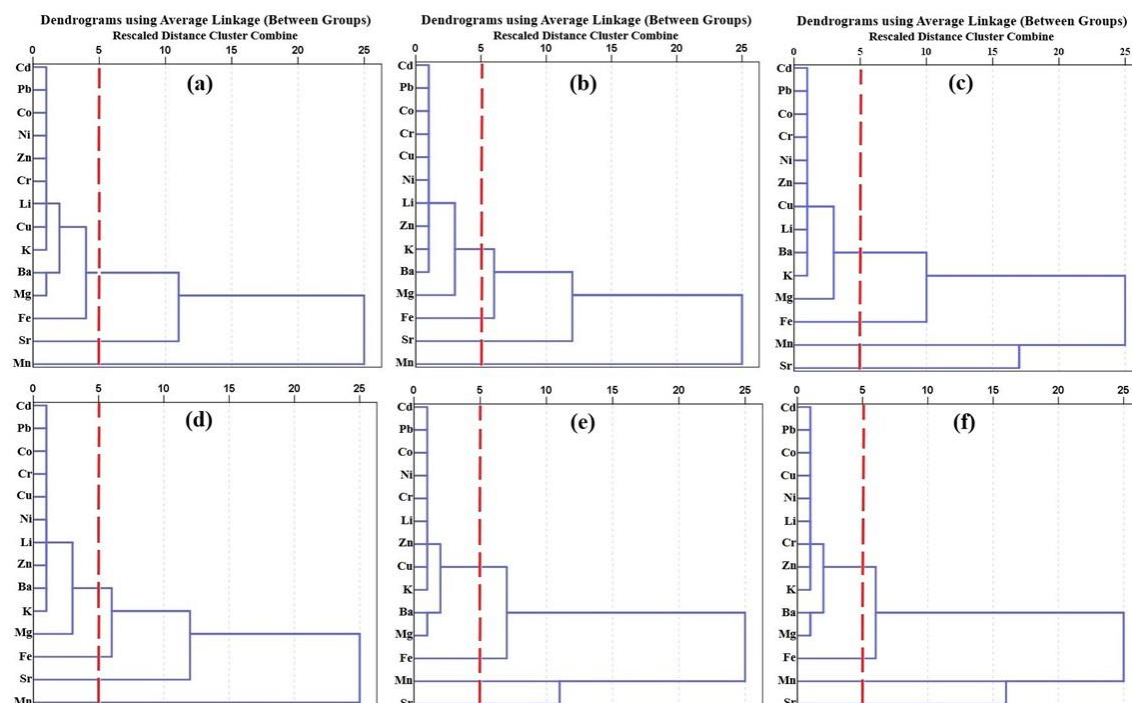
شکل ۸: طبقه‌بندی عناصر انتخابی (نسبت عناصر به کلسیم) در لایه‌های نمونه‌های صدف گردآوری شده از ایستگاه‌های نمونه‌برداری a: ایستگاه ۱، لایه پریماتیک، b: ایستگاه ۱، لایه نکرئوس، c: ایستگاه ۲، لایه پریماتیک، d: ایستگاه ۲، لایه نکرئوس، e: ایستگاه ۳، لایه پریماتیک، f: ایستگاه ۳، لایه نکرئوس)، بر اساس تجزیه و تحلیل خوشه‌ای سلسله مراتبی (HCA) و بر مبنای پیوند میانگین و فواصل اقلیدسی. خط چین‌های قرمز به منظور گروه‌بندی خوشه‌ها استفاده شده است.
